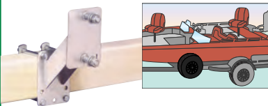
STC1000101 Pour support allant jusqu'à 3" x 4" Fits crossbar up to 3" x 4"
