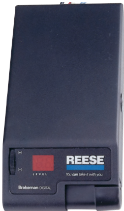
R83500 Pour remorques avec 2, 4, 6 ou 8 freins. Indicateur numérique. Compatible avec freins ABS For trailers with 2, 4, 6 or 8 brakes. Digital indicator. Compatible with ABS brakes.
