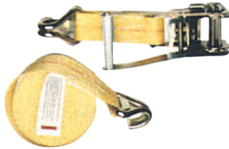
E51300 1" x 15' - 1,200 lb Noir / Black
