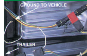
Faites la mise à terre Ground to vehicle
