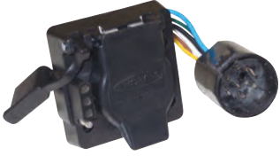
HP40955 Connecteur double/Double connector Ford / GM / Nissan Multi tow • 7/4 contacts
